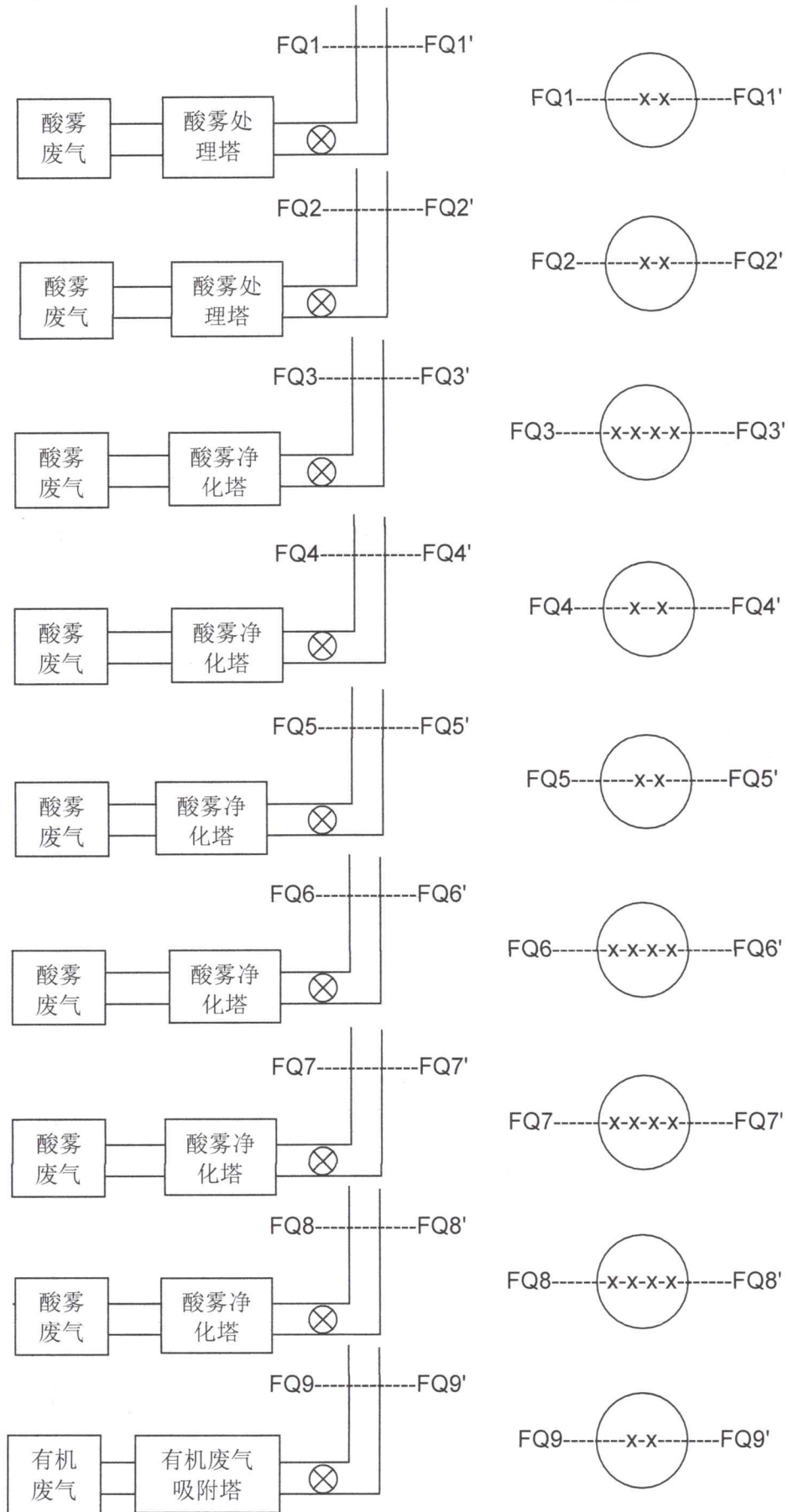
图 3 中国电子科技集团公司第二十六研究所废气有组织检测点示意图
