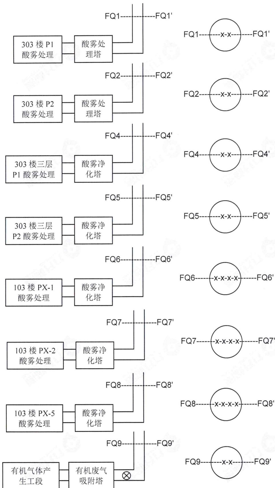
图 3 中国电子科技集团公司第二十六研究所废气有组织检测点示意图
